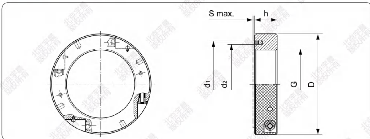
油脂驱动螺母部件图
